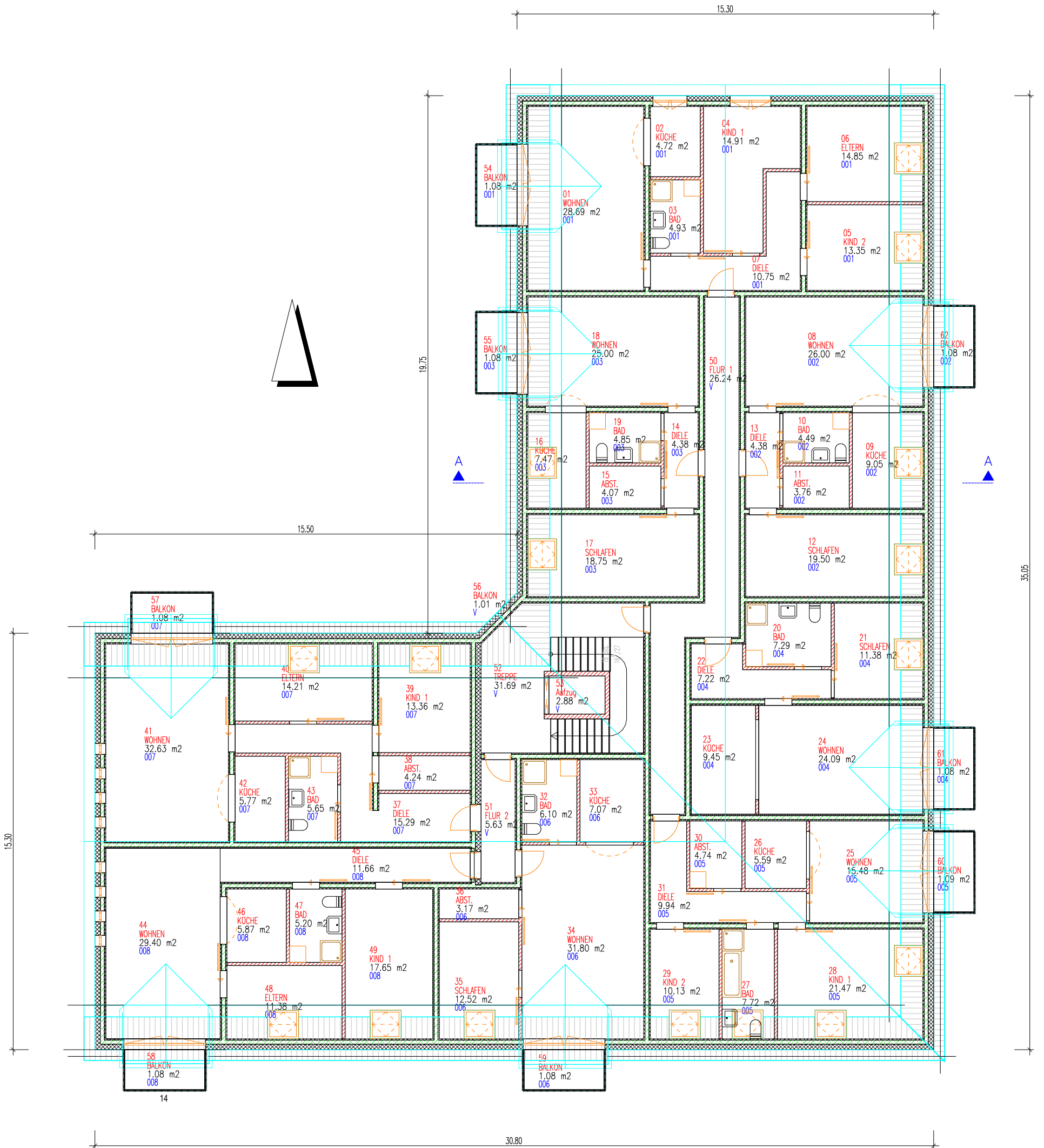
DACHGESCHOSS M 1:150
