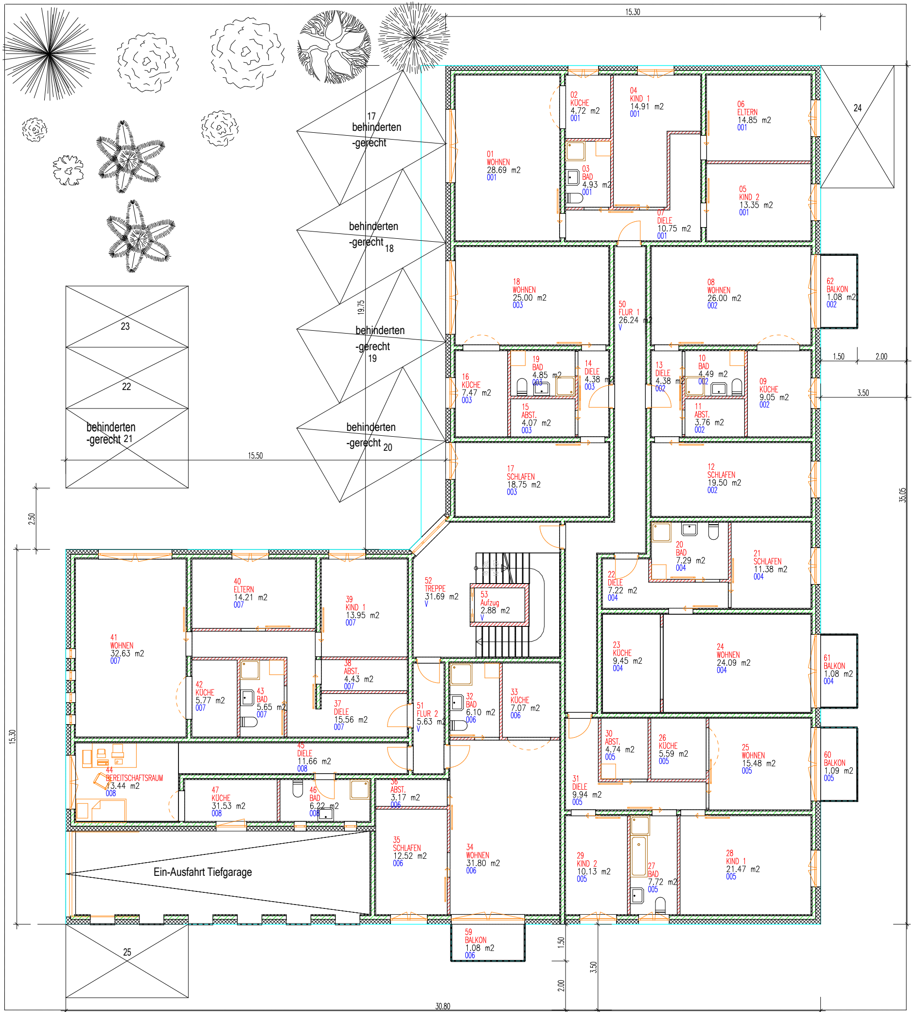
ERDGESCHOSS M 1:150
